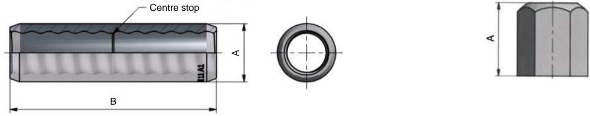
Bild 1: Kupplung, Mutter
